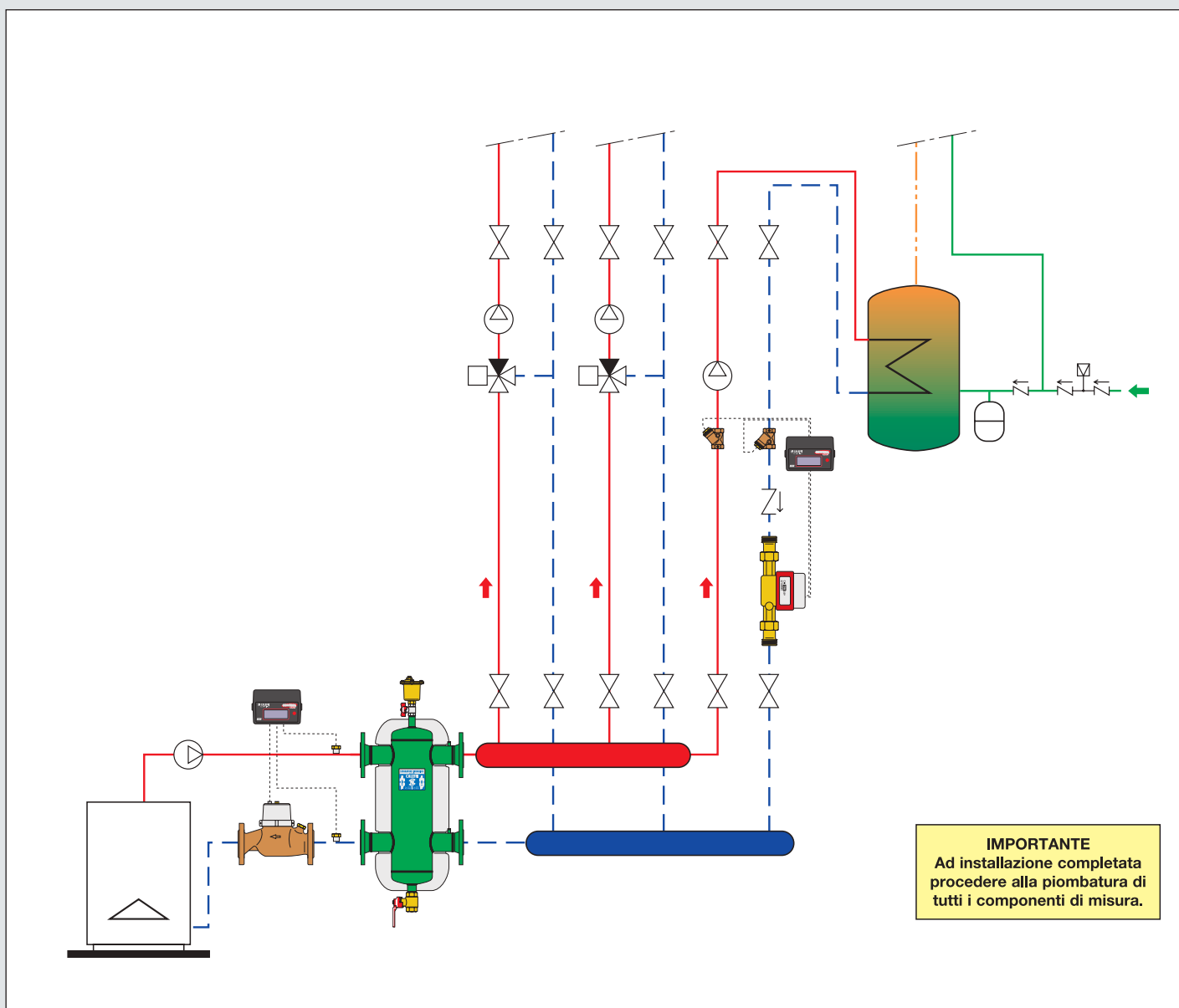
Schema indicativo di installazione
