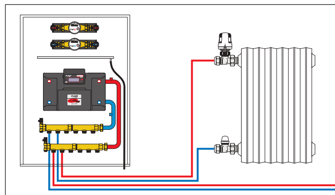
Schema applicativo distribuzione impianti a radiatori
